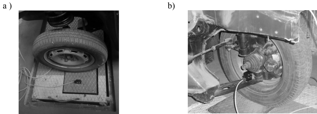
Fig. 10. Location of vibration acceleration sensors on the plate (a) and on the wheel (b) Rys. 10. Lokalizacja czujników przyspieszeń drgań na płycie (a) oraz na kole pojazdu (b)
