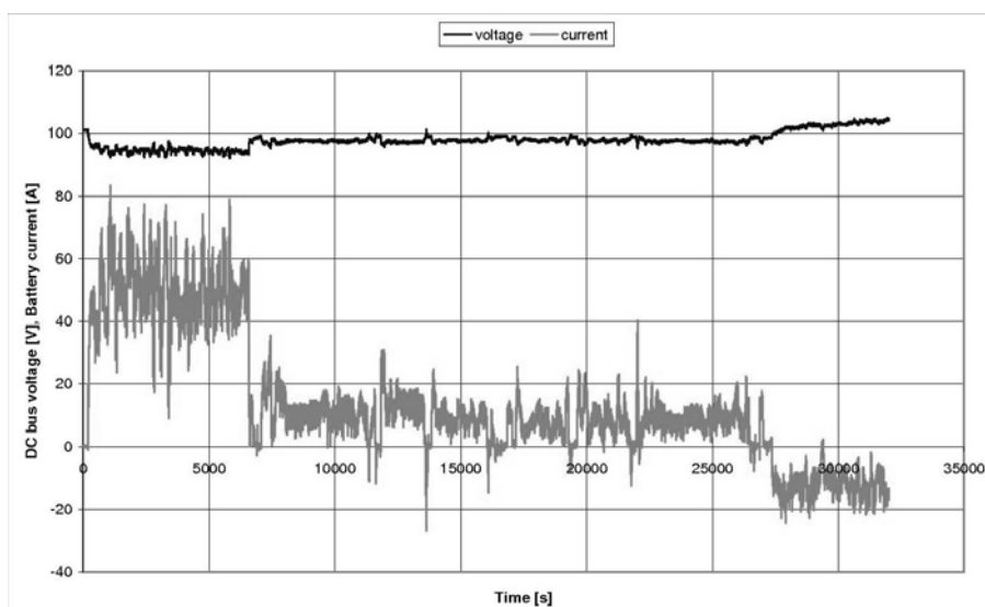
Fig. 7. DC bus voltage and battery current Bild 7. Gleichstromhauptleitung Spannung und Batterie Strom
