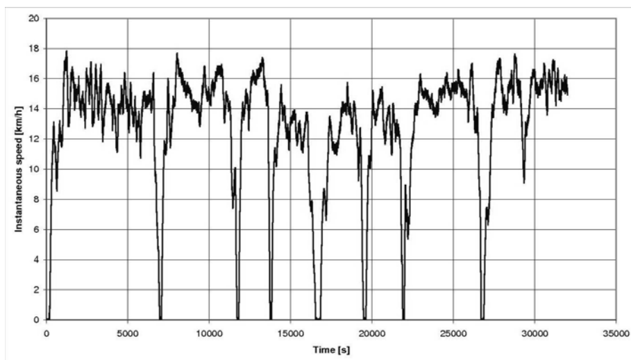
Fig. 6. Vehicle speed Bild 6. Geschwindigkeit des Fahrzeuges
