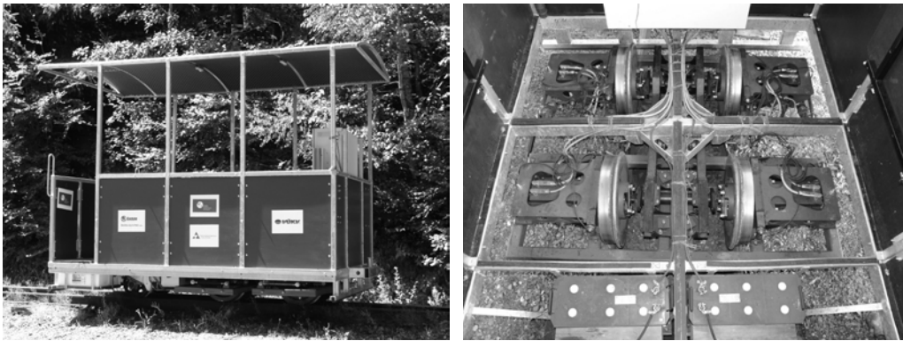
Fig. 3. Experimental vehicle at the railway line and bogie detail Bild 3. Experimentelle Fahrzeug an der Eisenbahnlinie und Fahrzeugchassis
