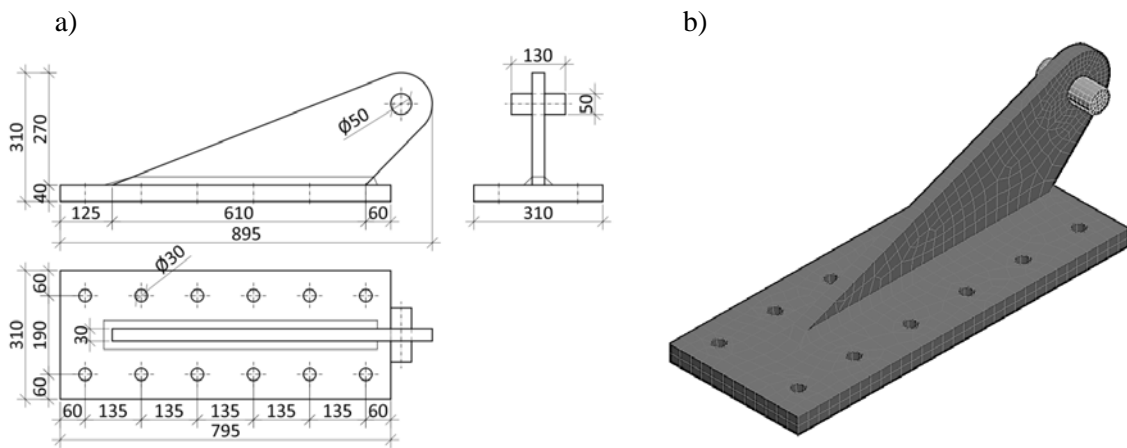
Fig. 4. The computational model of anchorage: a) geometry and dimensions; b) general view Rys. 4. Model obliczeniowy: a) geometria i wymiary; b) widok ogólny
